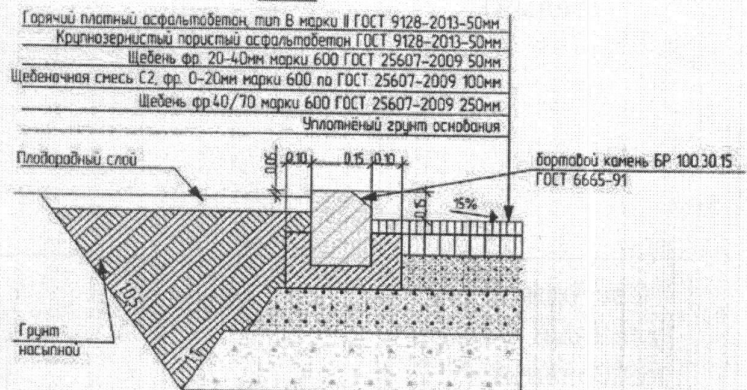
Схема дорожной конструкции Тип 11
