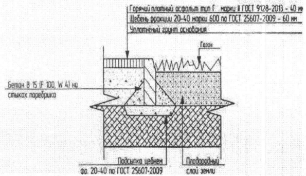
Узел конструкции пешеходной дорожки Тип 3
